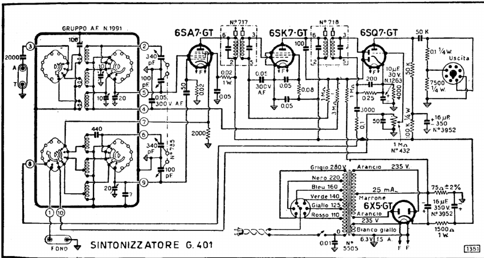
GELOSO - Sintonizzatore G 401 - Onde medie da 190 a 580 m. e due bande onde corte da 16 a 29 m. e da 29 a 53 m. Media frequenza 467 kc/s. Consumo 35 V/A.
